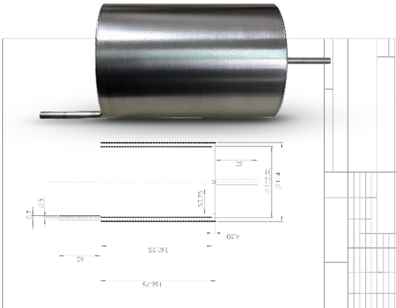
Doppelwandtiegel Double wall crucible
