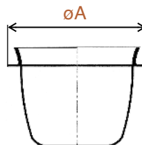
3 flacher Boden (für Claisse-Fluxer und Lego) 3 flat base (for Claisse-Fluxer and Leco)
